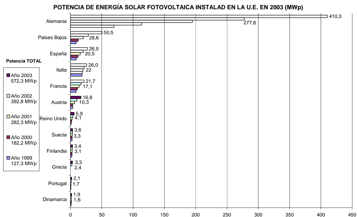
Figura 1. Potencia instalada por países en la U.E. Datos en MWp
