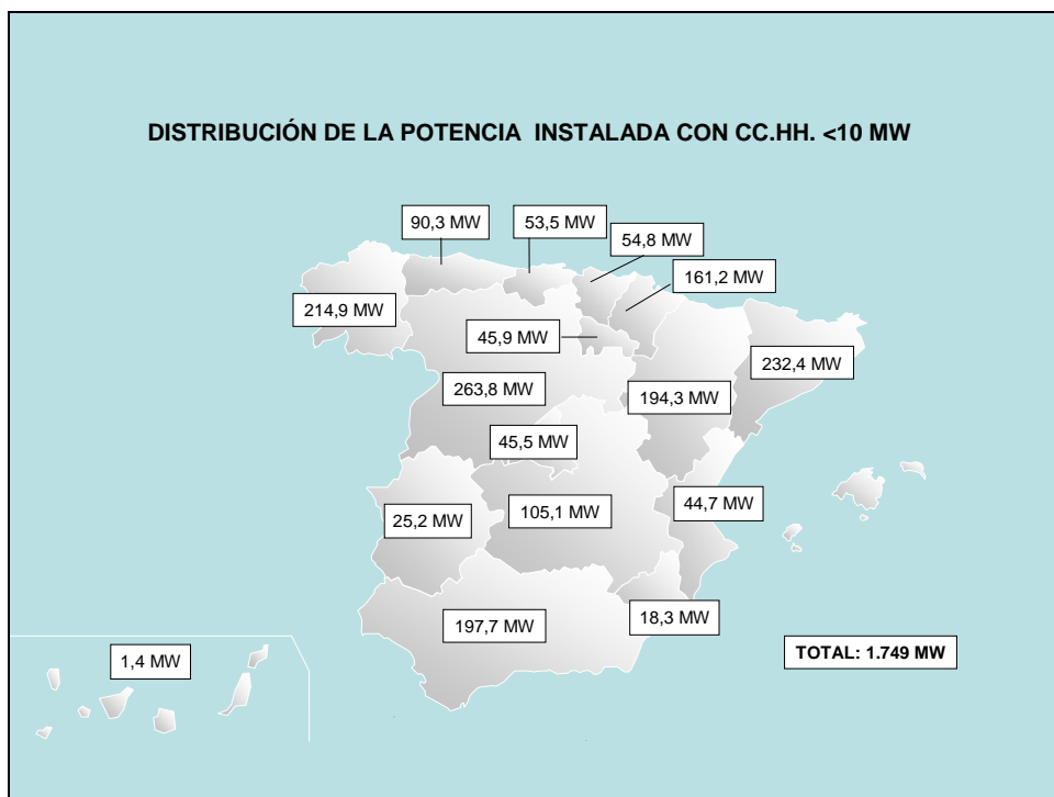
Figura 3.- Desglose por CC.AA de la potencia total acumulada con CC.HH menores de 10 MW a finales del 2004.
